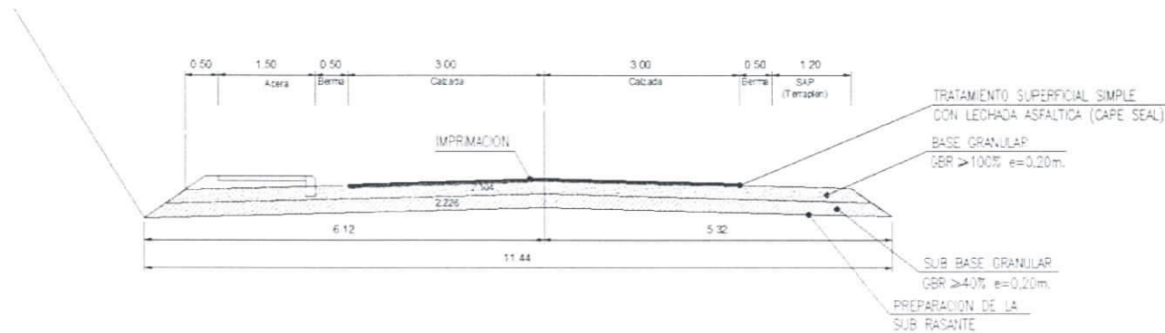
PERFIL TIPO 1 Dm. 0,000 a Dm. 0.437,069
