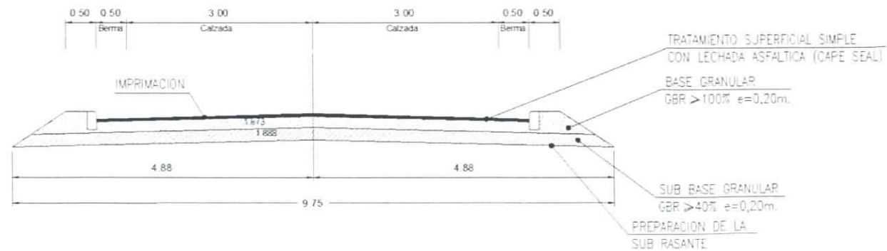
PERFIL TIPO 2 Dm 0.437,069 a Dm 1.260,000
