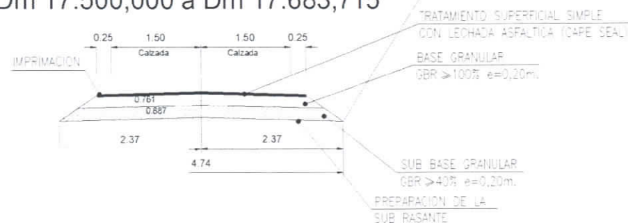
PERFIL TIPO 4 Dm 17.500,000 a Dm 17.683,715
