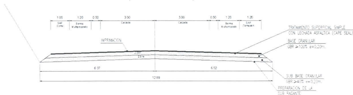
PERFIL TIPO 5 Dm 1.540,000 a Dm 17.500,000
